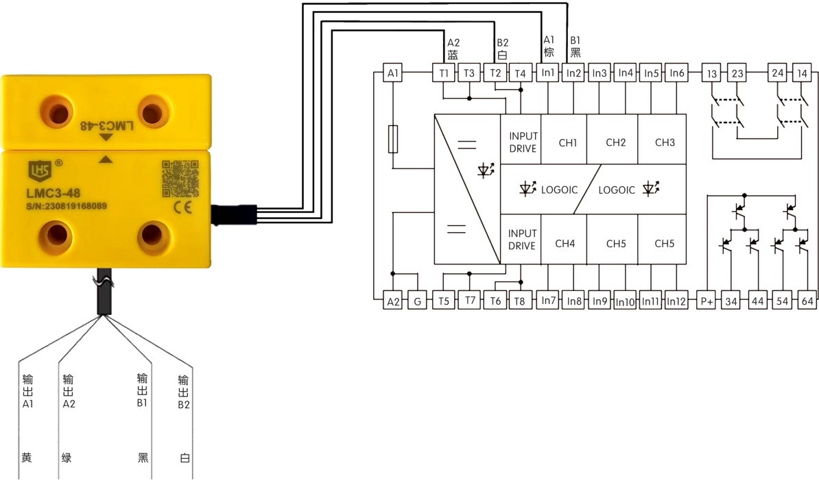
开关接线图（双路输出）
