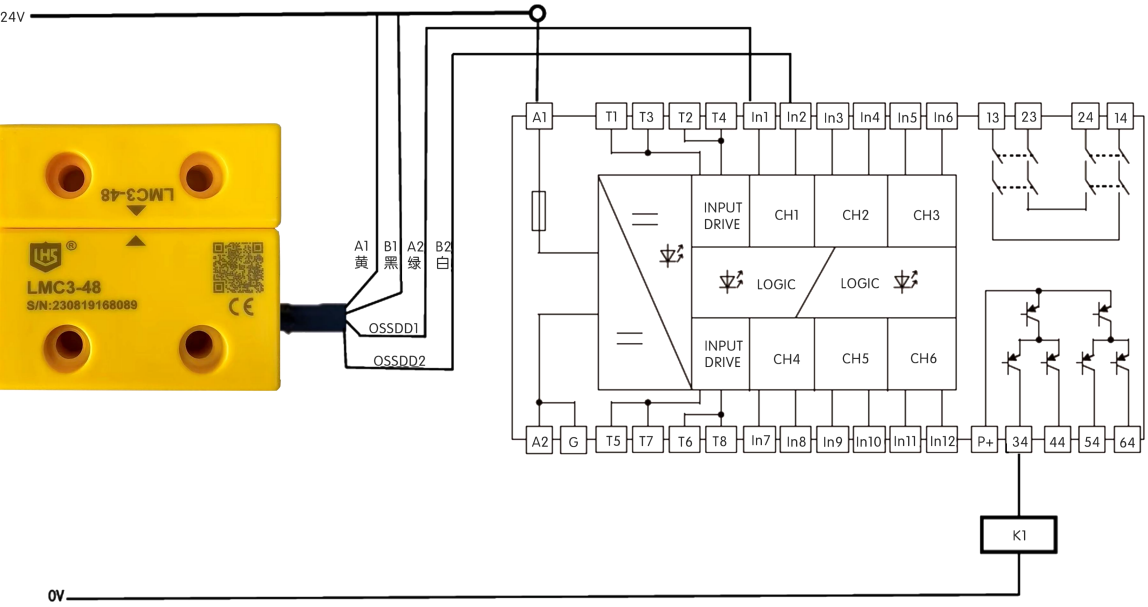
开关接线图（PNP双路输出）
